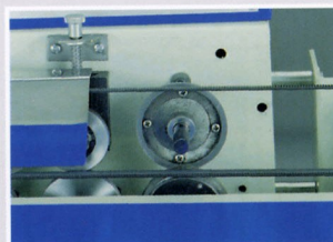
修邊器裝置封口後，將包裝袋殘餘邊切除。
